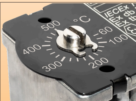
C: 螺丝刀的型号，带箭头和印刷的铝表盘，用于 JPCI 或其他供应商的 PPS Ex-c 外壳进行伴热；
