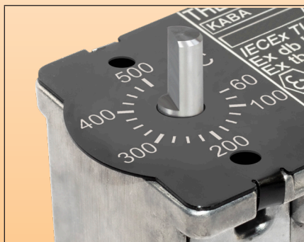
A: 轴直径6mm，长度10mm，用于印刷旋鈕和边框，或小塑料箭头旋鈕（可作为下面的配件提供）；
