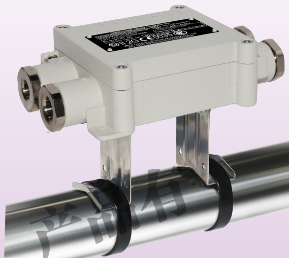
用型号为6YTQT的不锈钢支架隔开安装在管道上的示例
