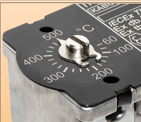
C: 螺丝刀的型号，带箭头和印刷的铝表盘，用于 JPCI 或其他供应商的 PPS Ex-e 外壳进行伴热；
